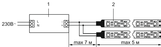
Рисунок 3 – Схема подключения одноцветной светодиодной ленты
